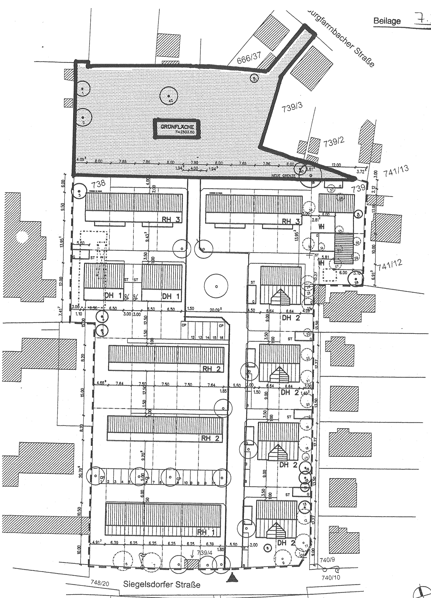
Erschließungs- und Bebauungskonzept ehem. Sportflächen an der Siegelsdorfer Straße Plan Nr. 3N-1-23-2003 vom 18.12.03
