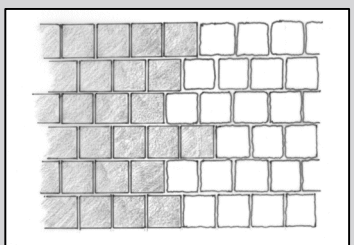
3. Verzahnung: Granitgroßsteinpflaster nicht gesägt und Granitgroßsteinpflaster gesägt, gestockt
