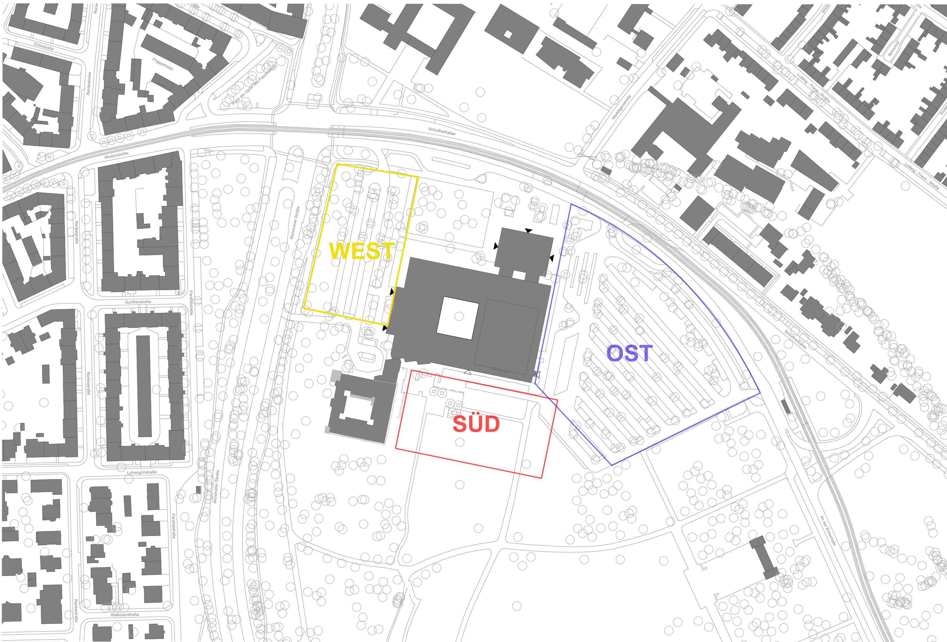
Anlage 1: Lageplan der Meistersingerhalle Nürnberg Verortungsmöglichkeiten M. 1:500
