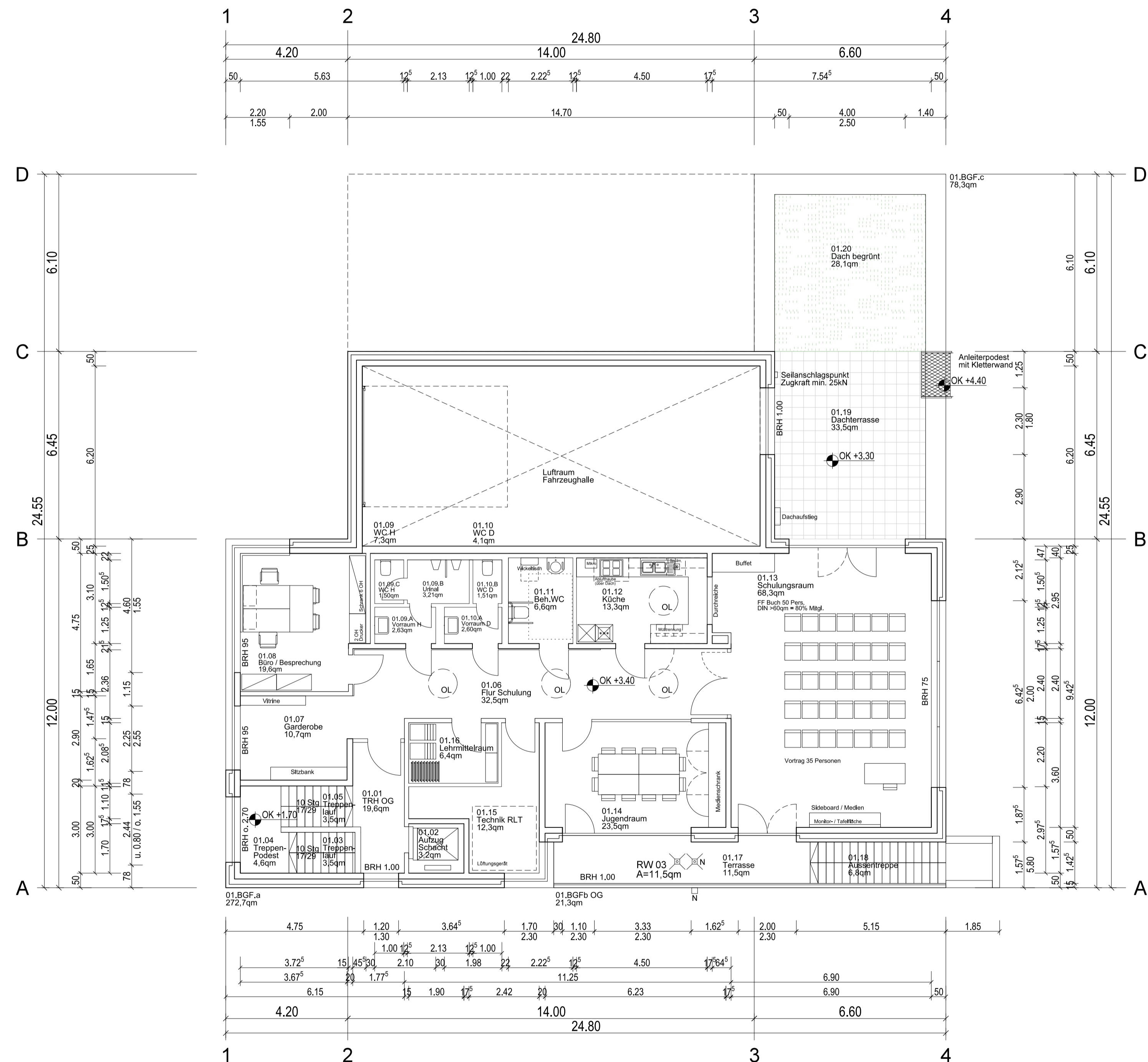
GRUNDRISS OG - M 1:100
